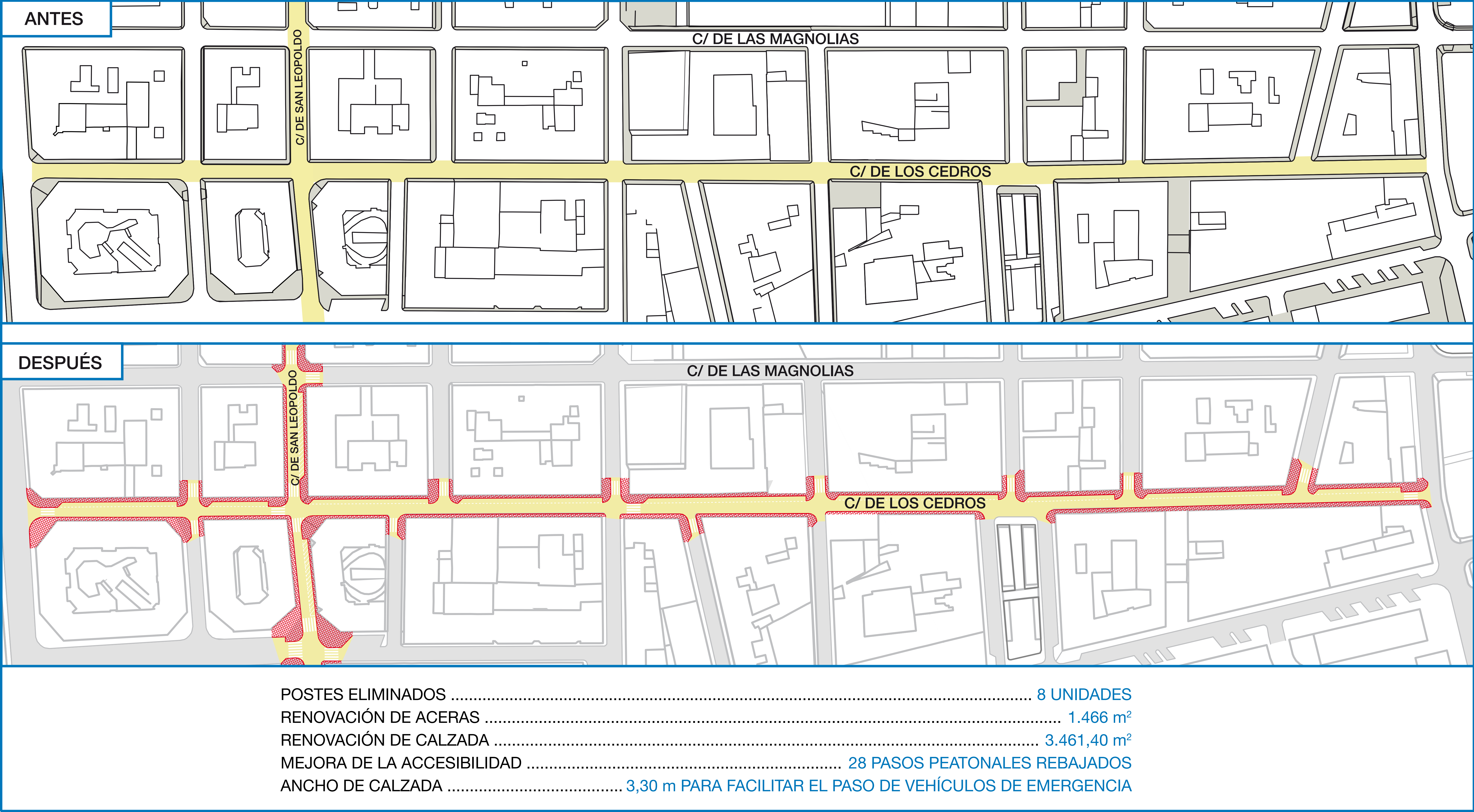
DETALLE PLANO PLANTA - CALLE DE LOS CEDROS
